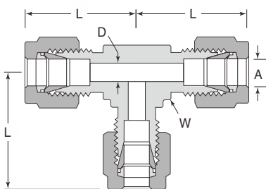
卡套三通中间接头(英制)
