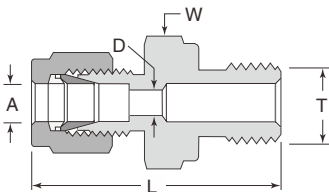
ISO/BSP平行外螺纹直通终端接头(英制)
