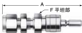
KC系列卡套穿板公头
